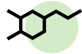
Dopamine
