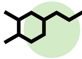
Dopamine
